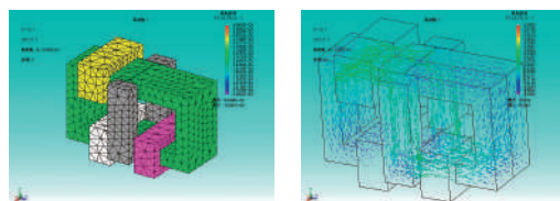
(a)磁心構成 (b)磁束密度分布
