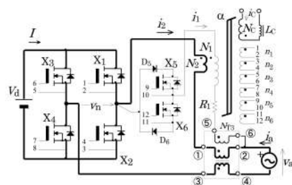
図2 磁気漏れトランスを付加したインバータの構成
