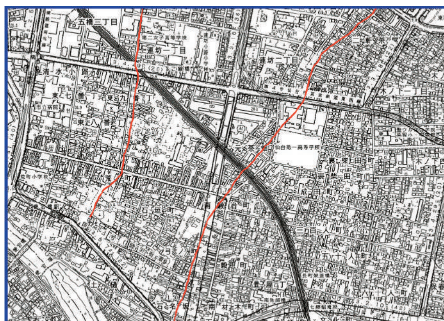
図4 調査範囲南部（連坊～広瀬川間）における活断層分布図
