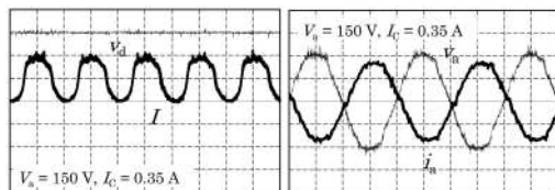
(a)入力側電圧電流 (b)出力側電圧電流
