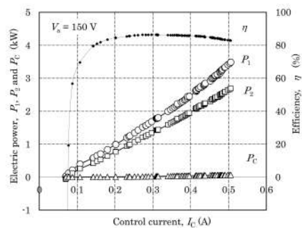
図7 入出力電力制御特性測定例
