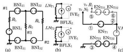
図3 磁気漏れトランスの SPICE モデル
